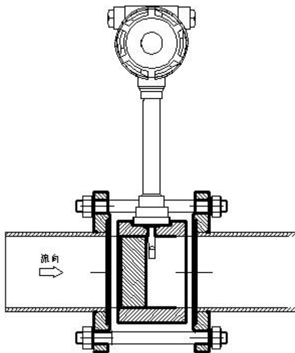
图二. 法兰夹装式结构图
